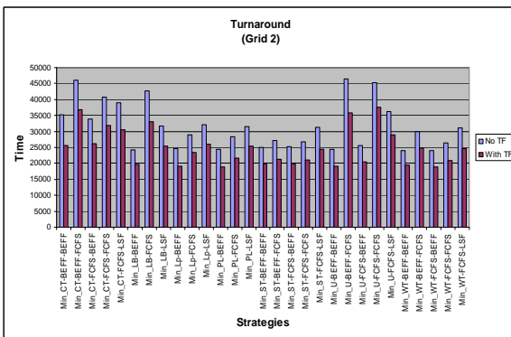
Figura. 10. Gráfica comparativa para la métrica Turnaround, Grid 2
