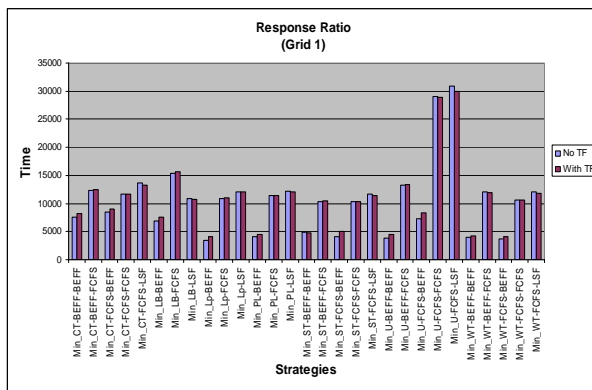
Figura 6. Gráfica comparativa para la métrica Response Ratio, Grid 1
