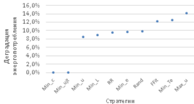
Рис. 10. Средняя деградация энергопотребления.
