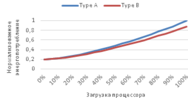
Рис. 5. Нормализованное энергопотребление задач типа А и В в зависимости от загрузки процессора (%).
