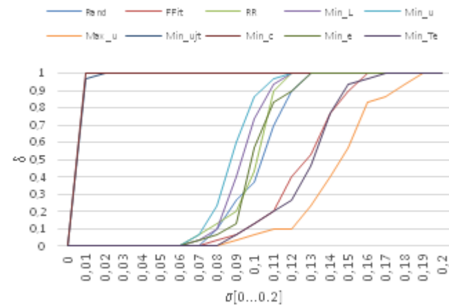
Рис. 11. Профиль деградации энергопотребления 10 стратегий.
