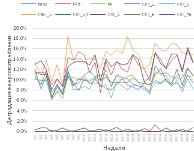
Рис. 9. Деградация энергопотребления по неделям.
