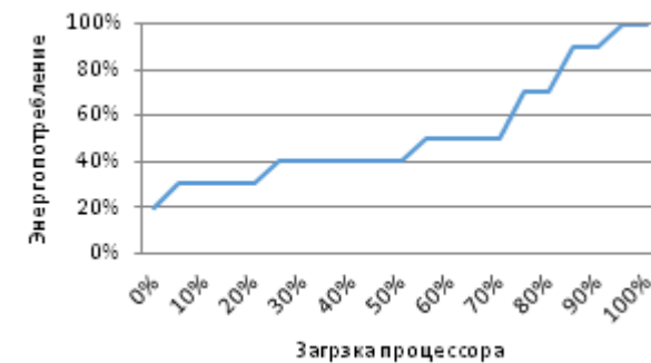
Рис. 2. Энергопотребление в зависимости от загрузки процессора (%).
